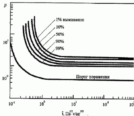
Рисунок 5-3. P-I диаграмма для экспресс-оценки поражения людей от взрыва ТВС при прохождении УВ с отражением (человек находится на открытом пространстве, волна распространяется сверху к земле или человек находится у вертикальной отражающей поверхности, волна распространяется вдоль земли и отражается от вертикальной поверхности)
