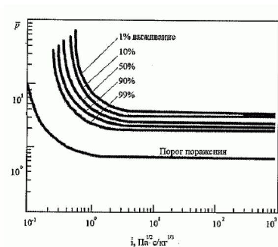
Рисунок 5-2. P-I диаграмма для экспресс-оценки поражения людей от взрыва ТВС при прохождении УВ без ее отражения (человек находится на открытом пространстве, волна распространяется вдоль земли)
