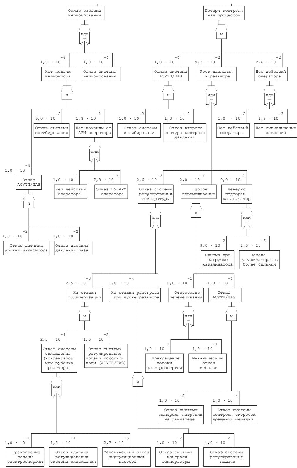
Рисунок 8-1. Пример дерева отказов для химических реакторов
