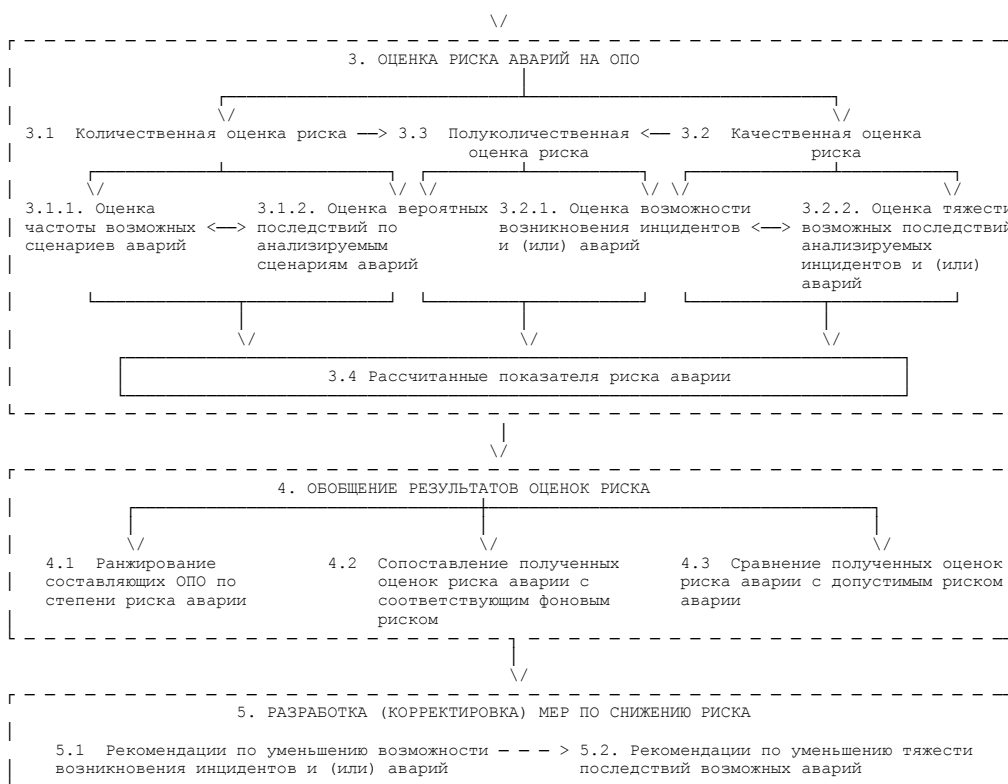
Рис. 2-1. Общая схема анализа опасностей и оценки риска аварий на ОПО
