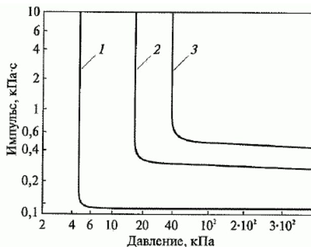
Рисунок 5-1. P-I диаграмма для оценки уровня разрушения промышленных зданий: 1 - граница минимальных разрушений; 2 - граница значительных повреждений; 3 - разрушение зданий (50 - 75% стен разрушено)
