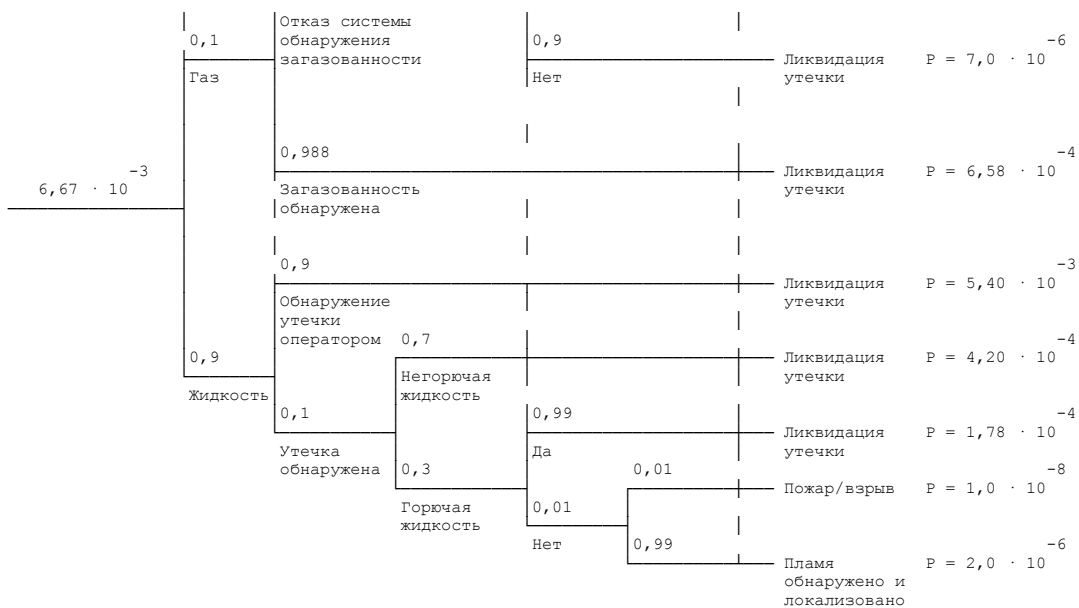
Рисунок 8-2. Пример дерева событий для случая разгерметизации сосудов, работающих под давлением
